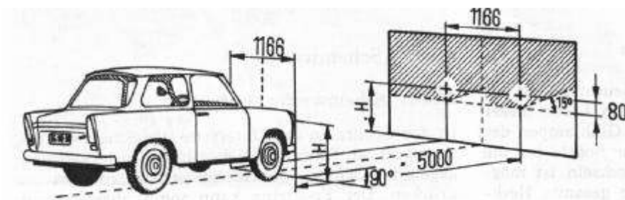
Bild E 25. Scheinwerfer einstellen
