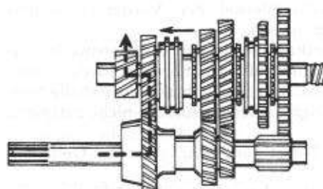
Bild G 6. Kraftverlauf für den 4. Gang
