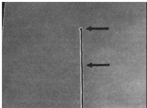
Bild K 8. Riß anbohren und anschrägen
